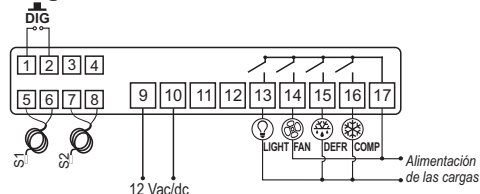
Imagen III - Conexión 12 Vac/dc
