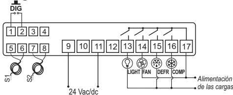
Imagen IV - Conexión 24 Vac/dc
