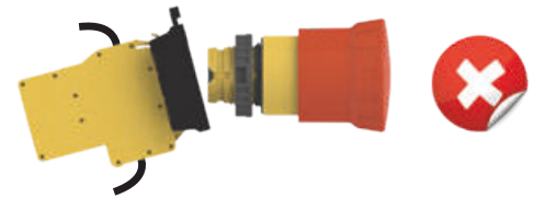
Brida NO montada correctamente en el botón.
