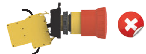
Bloque NO montado correctamente en la brida.
